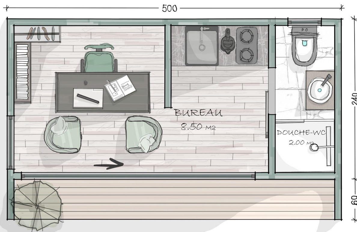
PLAN BUREAU-15- (15 m 2 )
